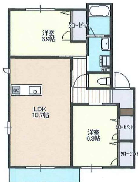
《間取り図》
